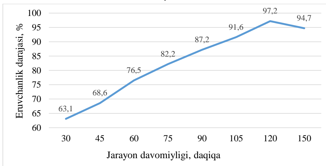
3-rasm. Oltinning eruvchanlik darajasining jarayon davomiyligiga va shox arog‘i konsentratsiyasiga bog‘liqligi
